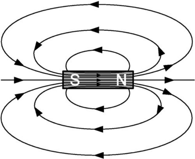
Fig. 5.46 Bar magnet
