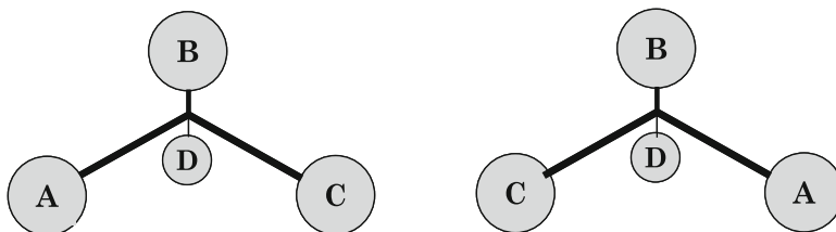
Fig. 8.65 Enantiomorphs
