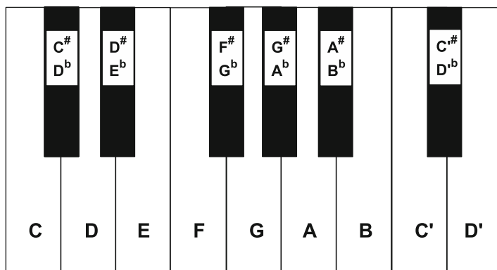
Fig. 2.32 Piano keyboard
