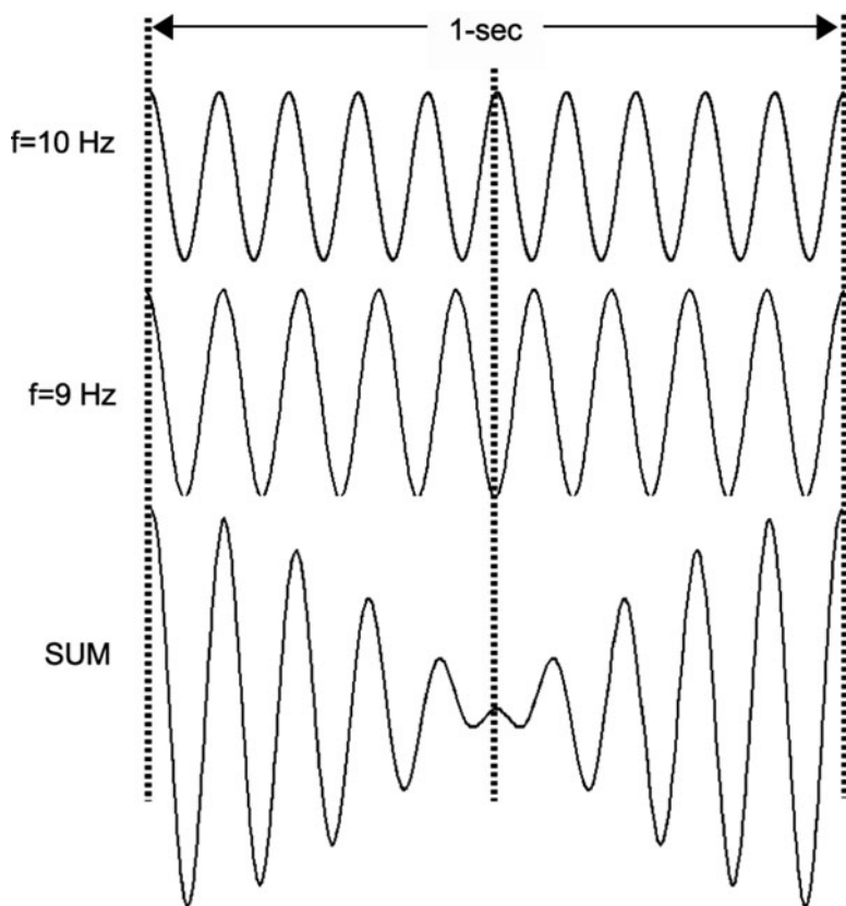
Fig. 7.16 Beats
