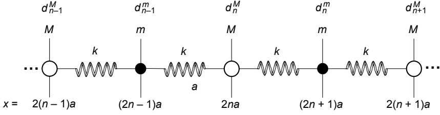
Fig. 2.4. The diatomic linear lattice
