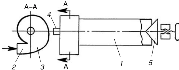
Fig. 2.20. A vortical tube
