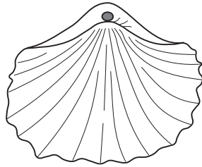
Rhynchonellida
