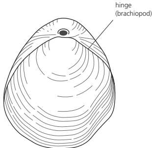
Hinge
