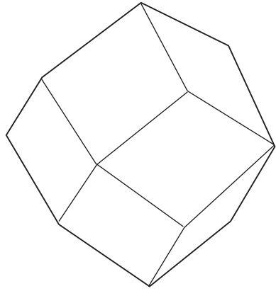
Cubic
