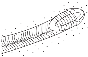
Cruziana
