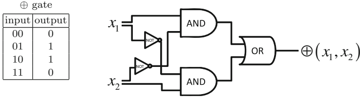
Fig. 3.1 Exclusive OR \oplus
