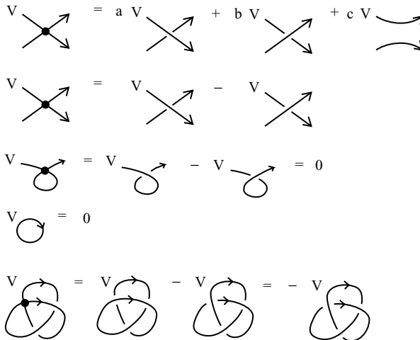
Fig. 16. Graphical vertex formulas.
