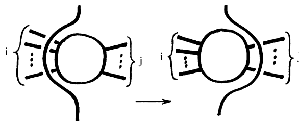
Fig. 10. The (i, j) -pass move.
