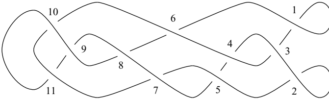
Fig. 30. The Legendrian knots L .
