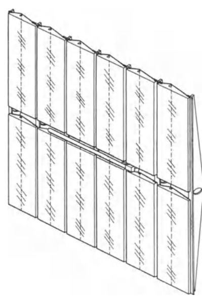
Fig. 2 Heliostat Type II
