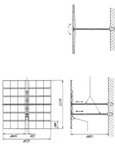
Fig. 2 Heliostat Type II
