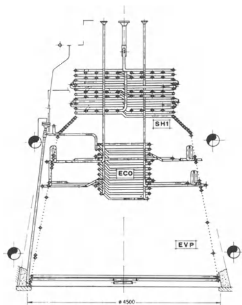
FIG. 1 - SEZIONE DELLA CALDAIA
