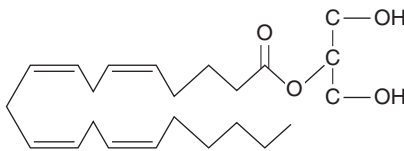
2-Arachidonoyl glycerol (2-AG)
