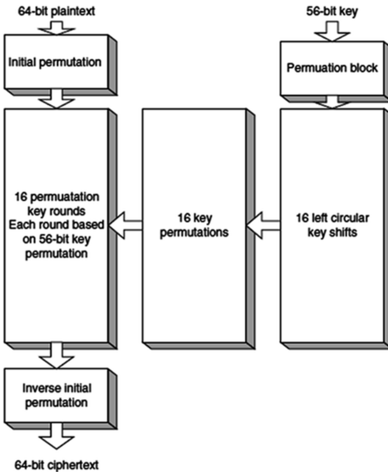
Fig. 11.3 DES algorithm
