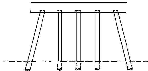
Fig. 6.7.2-Pile bent
