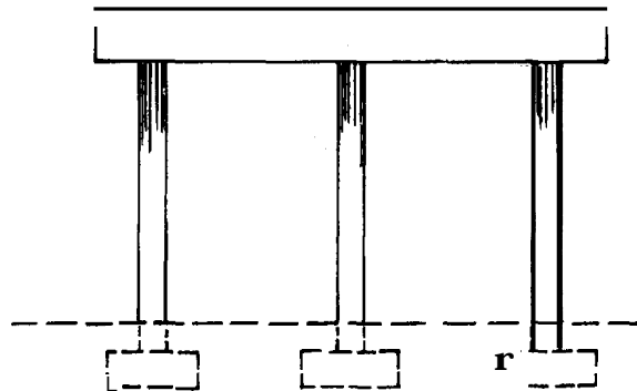
Fig. 6.7.3-Multi-column bent
