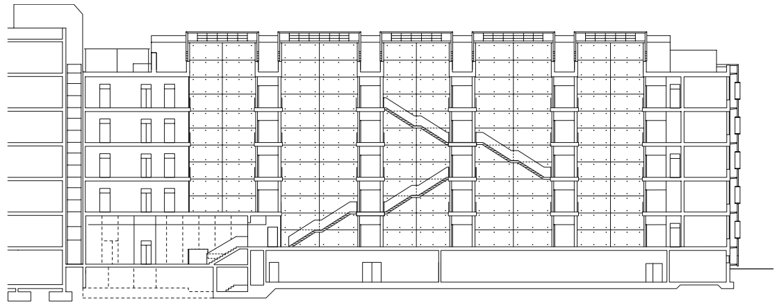
Longitudinal section
