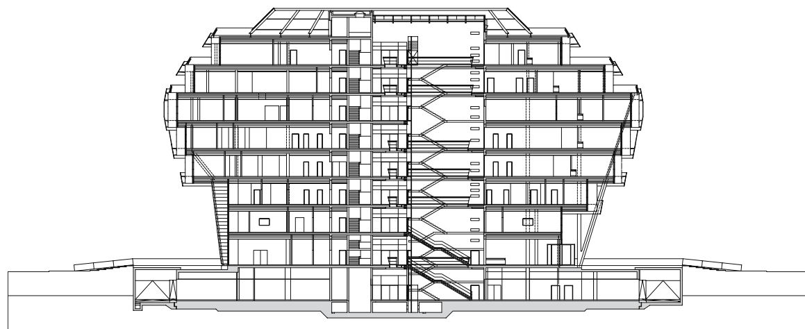
Longitudinal section
