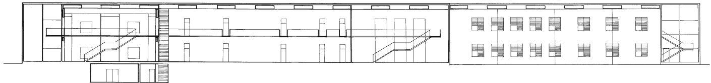
Longitudinal section
