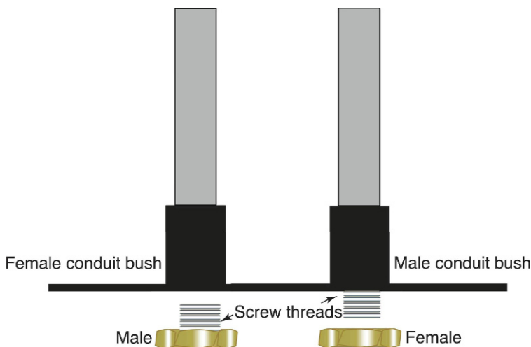
FIGURE 2.38 Conduit termination.
