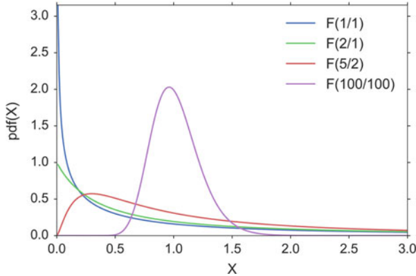
Fig. 6.16 F -distribution
