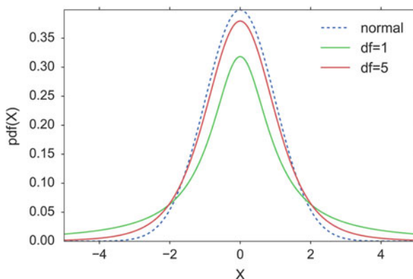
Fig. 6.13 t -Distribution
