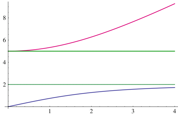
Fig. 4.1 Optical eigenmodes
