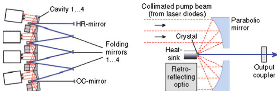
Fig. 7.36 The Trumpf 4 kW thin disk DPL
