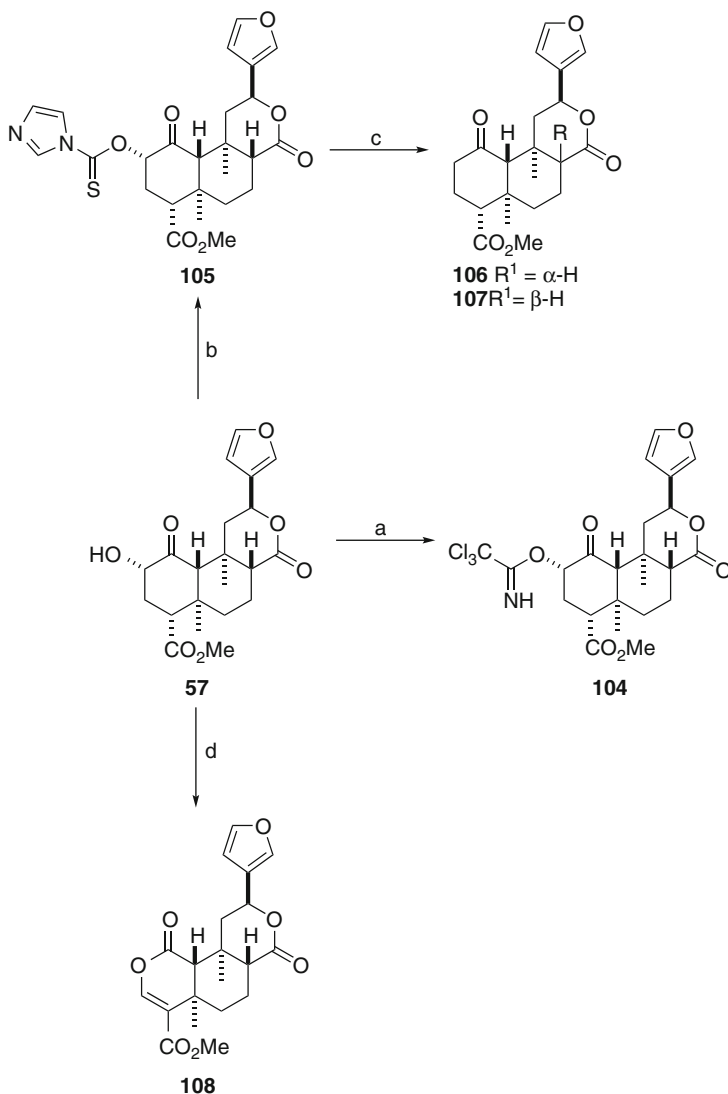
Scheme 16 (a) Trichloroacetoneitrile, DBU, \text{ClCH}_2\text{CH}_2\text{Cl} , 0^\circ\text{C} ; (b) (\text{Im})_2\text{CS} , DMAP, \text{CH}_2\text{Cl}_2 ; (c) AIBN, \text{Bu}_3\text{SnH} , toluene; (d) \text{CrO}_3 , pyridine
