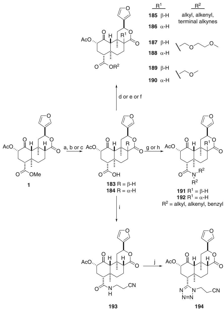
Scheme 28 (a) LiSEt, DMPU, 55 °C; (b) Ac 2 O, DMAP, pyridine; (c) LiI, pyridine, 120 °C; (d) ROH, DCC, DMAP, CH 2 Cl 2 ; (e) MEMCl, i -Pr 2 NEt, CH 2 Cl 2 ; (f) MOMCl, Et 3 N, CH 2 Cl 2 ; (g) EDCl, HOBT, Et 3 N, DMF; (h) EDCl, DMAP, DMF; (i) 3-aminopropanenitrile, EDCl, HOBT, DMF; (j) PPh 3 , TMSN 3 , DIAD, THF
