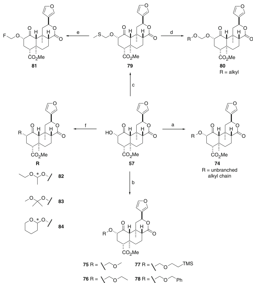
Scheme 10 (a) \text{RX} , \text{Ag}_2\text{O} , \text{CH}_3\text{CN} ; (b) \text{ROCH}_2\text{Cl} , i\text{-Pr}_2\text{NEt} , DMF; (c) \text{Ac}_2\text{O} , \text{AcOH} , \text{Me}_2\text{SO} ; (d) NIS, ROH, TfOH, 4-Å sieves; (e) NIS, \text{Et}_2\text{NSF}_3 , 4-Å sieves; (f) PPTS or PTSA, \text{CH}_2\text{Cl}_2
