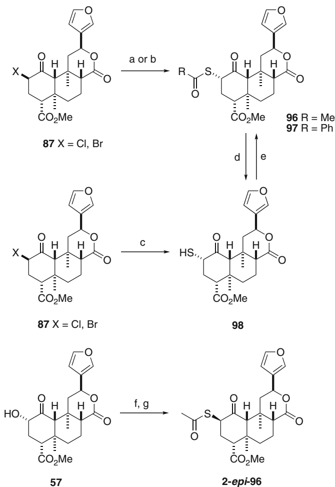
Scheme 14 (a) RCOSh, CH 3 CN; (b) potassium thioacetate, acetone; (c) NaSH, MeOH, DMF; (d) NaSMe, MeOH, CH 2 Cl 2 , -20\text{ }^{\circ}\text{C} ; (e) Ac 2 O, DMAP, CH 2 Cl 2 ; (f) (CF 3 SO 2 ) 2 O, pyridine, CH 2 Cl 2 , -20\text{ }^{\circ}\text{C} ; (g) potassium thioacetate, acetone, -20\text{ }^{\circ}\text{C}
