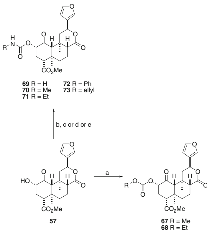
Scheme 9 (a) Chloroformate, DMAP, CH 2 Cl 2 ; (b) Cl 3 C(O)NCO, CH 2 Cl 2 ; (c) Al 2 O 3 ; (d) appropriate isocyanate, DMAP, pyridine; (e) appropriate isocyanate, TMSCl, CH 2 Cl 2
