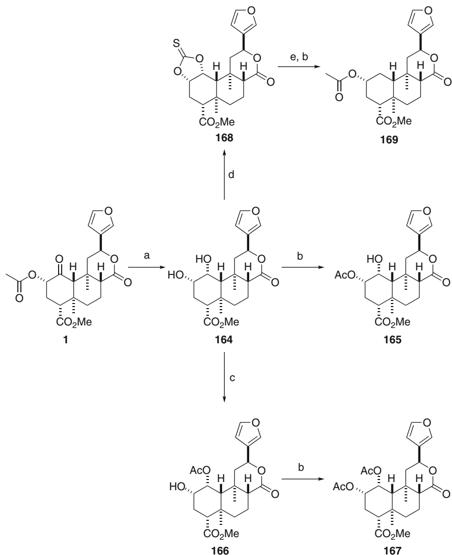
Scheme 26 (a) \text{NaBH}_4 , i -PrOH; (b) \text{Ac}_2\text{O} , pyridine; (c) trimethyl orthoacetate, AcOH (cat.), 100^\circ\text{C} ; (d) thiocarboxydimidazole, DMF, 90^\circ\text{C} ; (e) \text{Bu}_3\text{SnH} , AIBN, toluene, 80^\circ\text{C}
