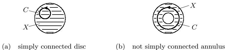
Fig. 5.12. Connectivity
