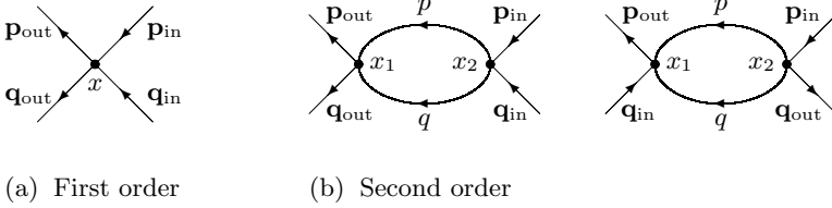
Fig. 15.2. Feynman diagrams
