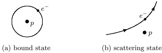
Fig. 2.11. Hydrogen atom
