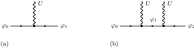
Fig. 1.2. Feynman diagrams
