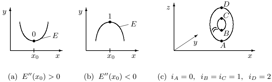
Fig. 5.19. Morse index
