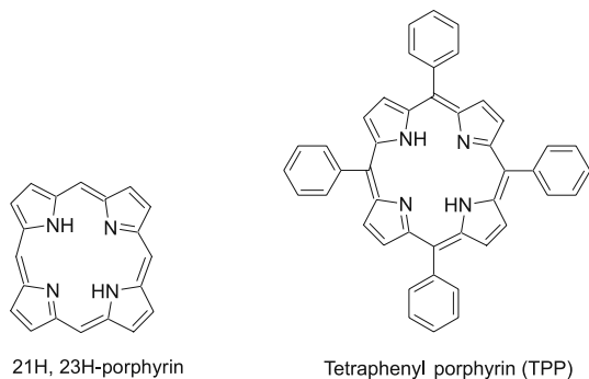
21H, 23H-porphyrin
