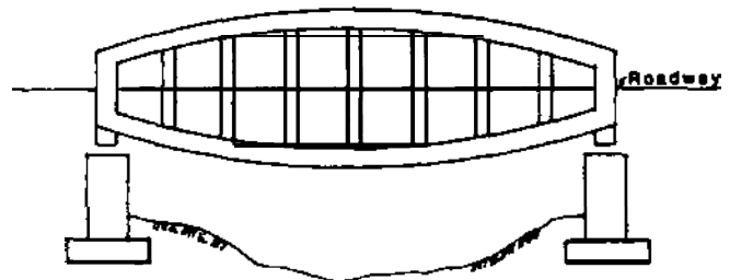
Fig. 2.5.6.1—Vierendeel truss bridge
