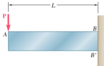
Fig. 6.34 ( PL \leq M_Y )
