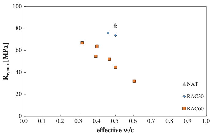
Fig. 7.21 w/c_{eff} - R_{c,max}
