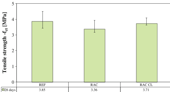
Fig. 5.9 Tensile strength
