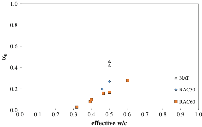
Fig. 7.22 w/c_{eff} - \alpha_0
