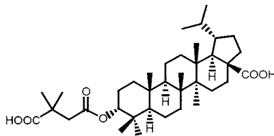
72 DSD
