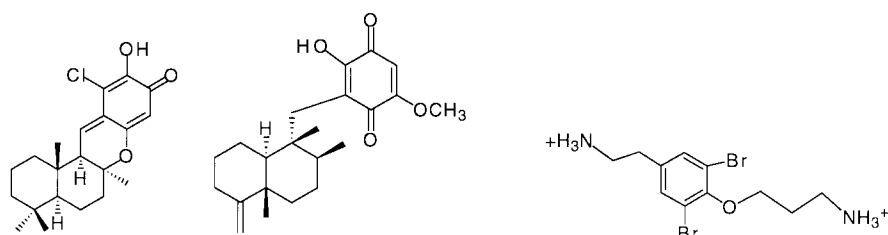
Chloropuupehenone (11)
