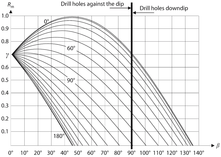
Fig. B2. \alpha = 45^\circ
