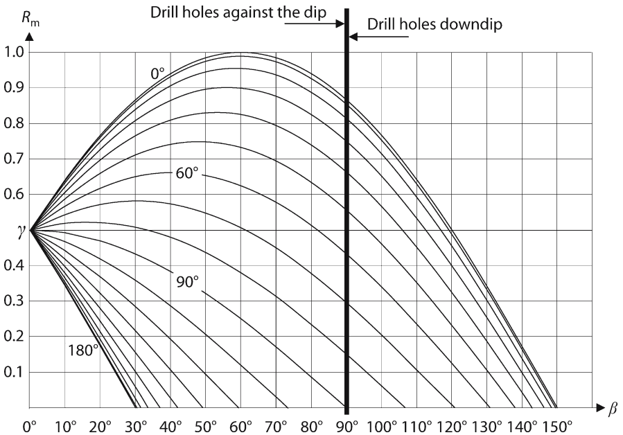
Fig. B1. \alpha = 30^\circ
