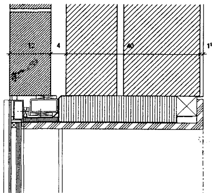
Fig. 57: Plan, 1:10
