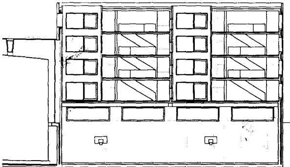
Fig. 159: Longitudinal section, 1:500
