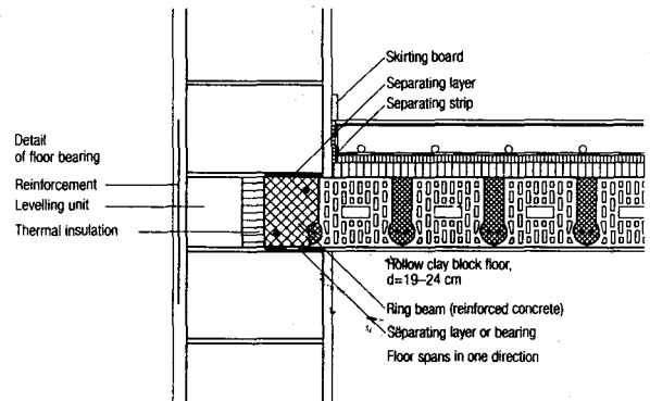
Longitudinal section
