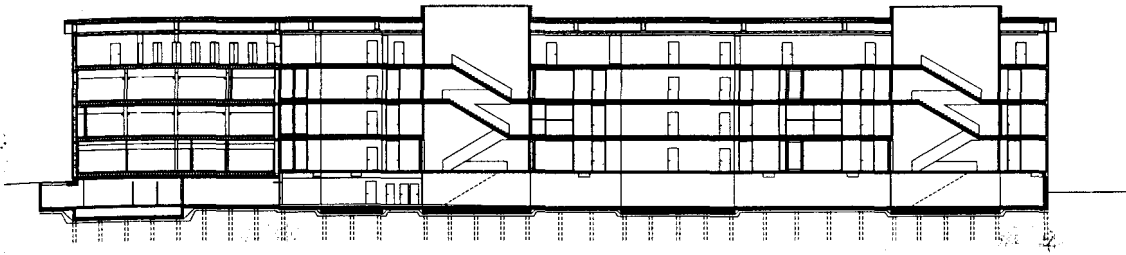
Fig. 262: Longitudinal section C-C
