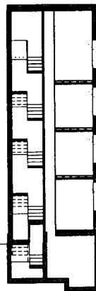
Fig. 289: Section
