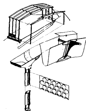
Fig. 53: Details of loadbearing construction Jean Prouvé: Pavillon du centenaire de l'aluminium, Paris (F), 1954
