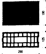
SwissModul® brick 125 mm
