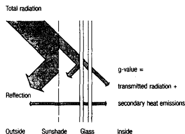
Fig. 74: External sunshade
