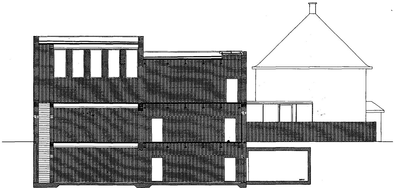
Fig. 73: Longitudinal section, 1:200
