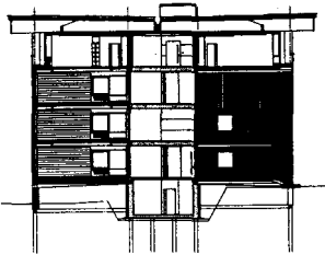
Fig. 263: Section A-A
