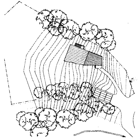
Fig. 287: Site plan
