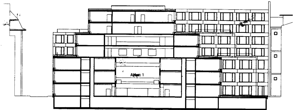
Fig. 189: Longitudinal section, 1:600
