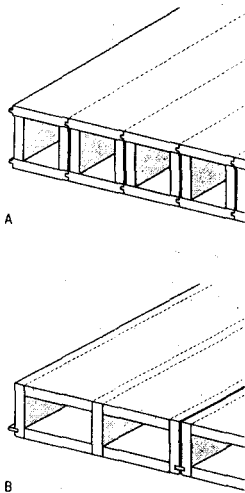
Fig. 33: Lignatur elements A) Box element B) Planar element
