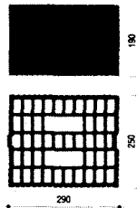
SwissModul® brick 250 mm
