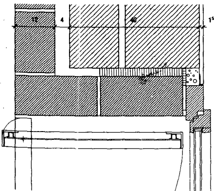
Fig. 54: Plan, 1:10
