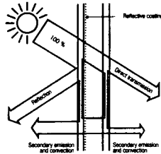
Fig. 254: Shading – the radiation relationship Source: "Glas und Praxis", Glas Trösch AG, 2000
