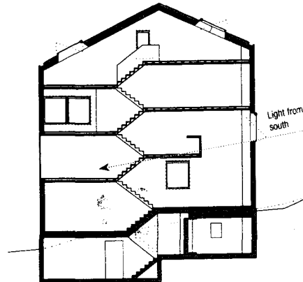
Fig. 294: Longitudinal section
