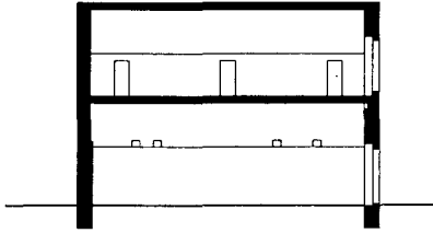
Fig. 61: Ghorfa type A Longitudinal section, 1:200
