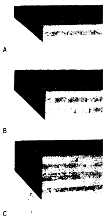
Fig. 27: LenoTec A) 3-ply, 81 mm B) 5-ply, 135 mm C) 7-ply, 216 mm
