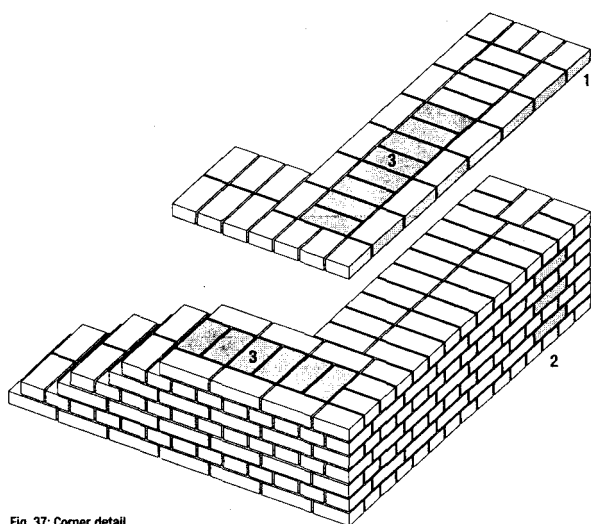
Fig. 37: Corner detail
