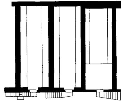
Fig. 70: Ghorfa type B Plan, 1:200
