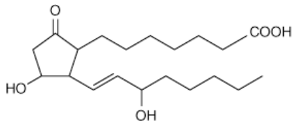
Alprostadil (prostaglandin E 1 )
