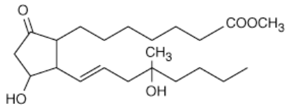
Misoprostol (prostaglandin E 1 analog)
