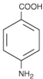
p-Aminobenzoic acid (PABA)
