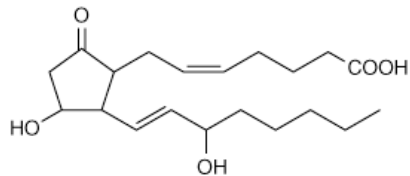
Dinoprostone (prostaglandin E 2 , PGE 2 )
