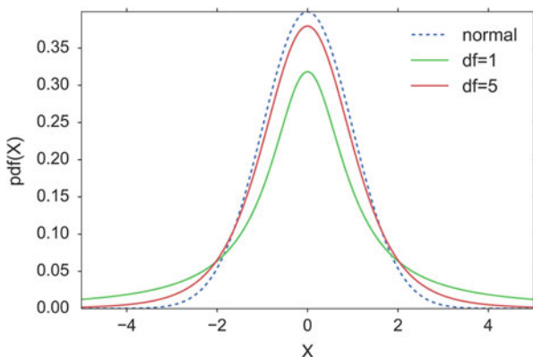
Fig. 6.13 t -Distribution
