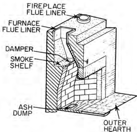
fireplace
