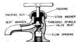
faucet
