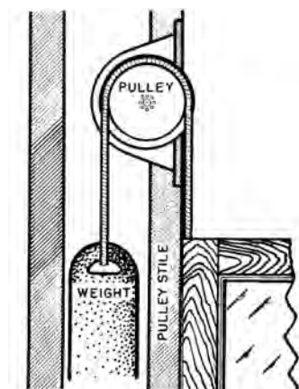
pulley stile
