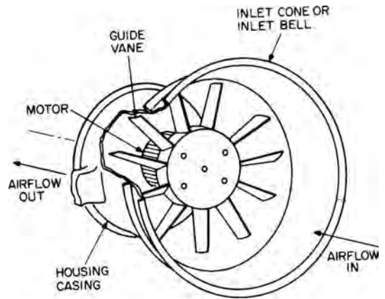
axial-flow fan
