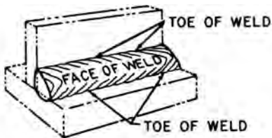
fillet weld
