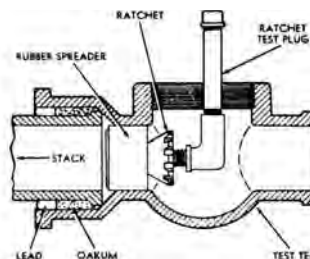
test tee
