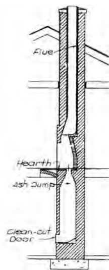
chimney
