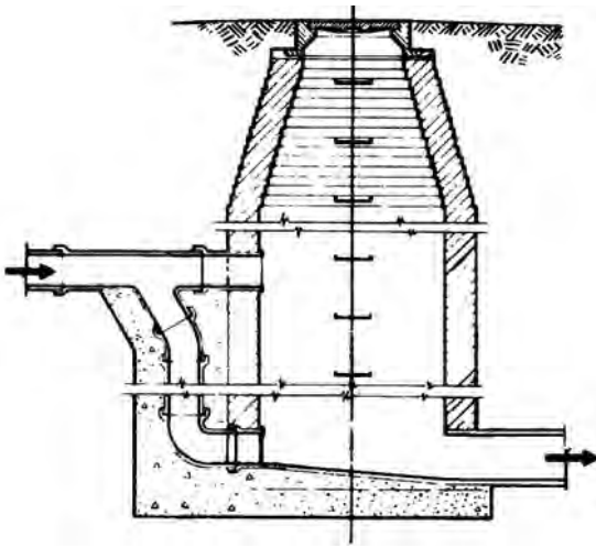
manhole
