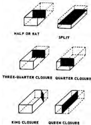
brick: nomenclature
