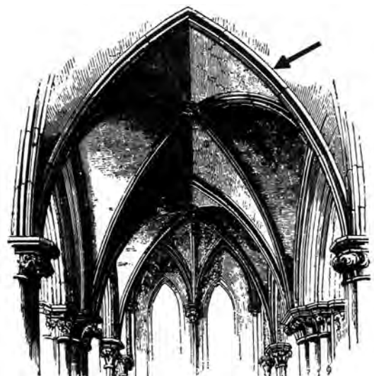
transverse rib
