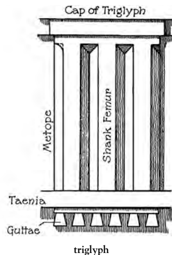
triglyph
