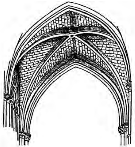
quadripartite vault
