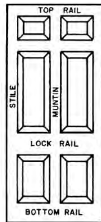
door nomenclature
