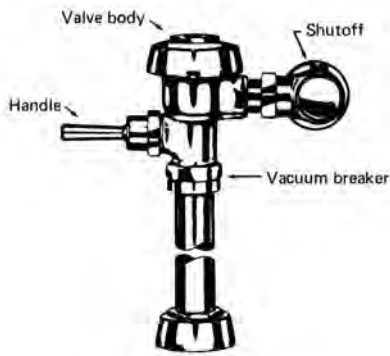
flushometer
