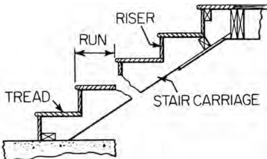
stair: nomenclature
