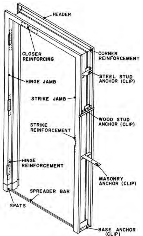
doorframe
