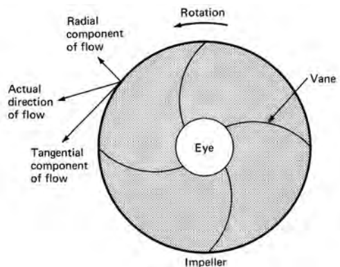
impeller
