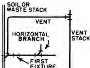
relief vent
