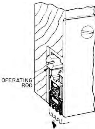
automatic door bottom
