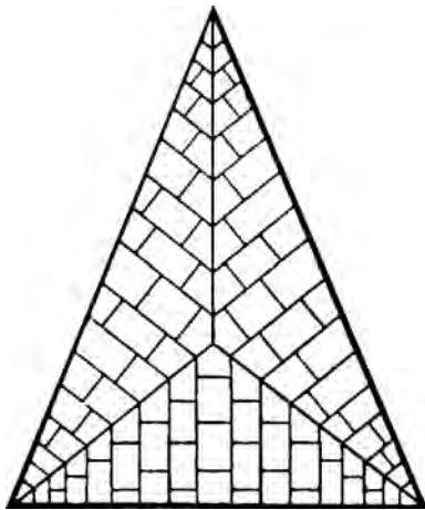
tripartite vault
