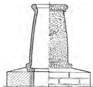
chimney pot
