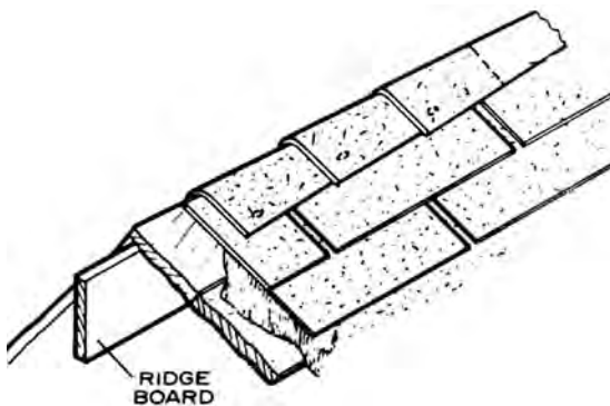
ridgeboard
