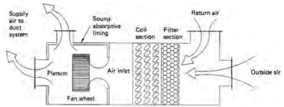
plenum fan
