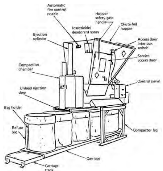
linear packer
