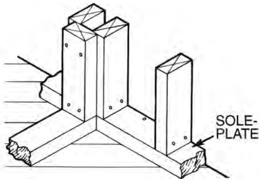
soleplate, 2
