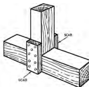
scab
