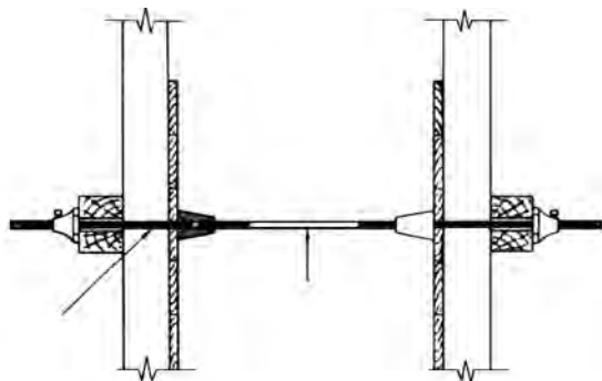
tie rod
