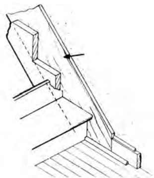
face string
