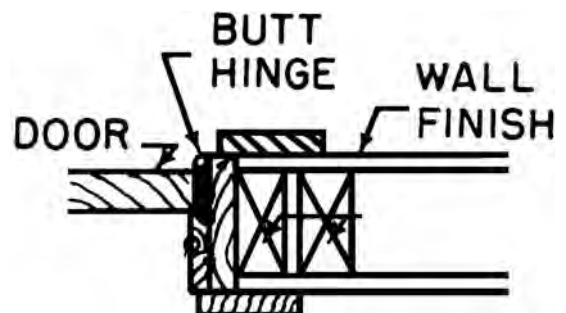
hinge jamb
