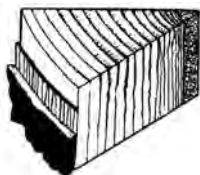
cambium
