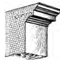
corona
