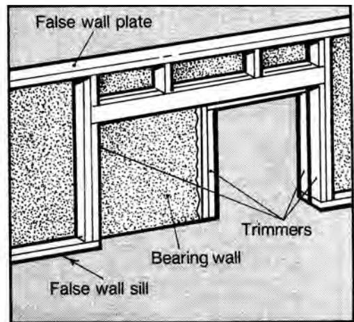
trimmer
