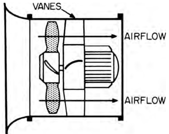
vaneaxial fan
