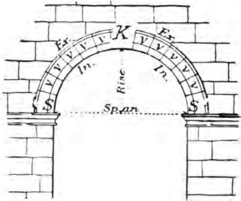
arch: Ex Estrados; In intrados; K keystone; S springers; v voussoirs
