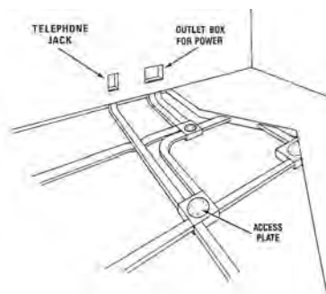
underfloor conduit system
