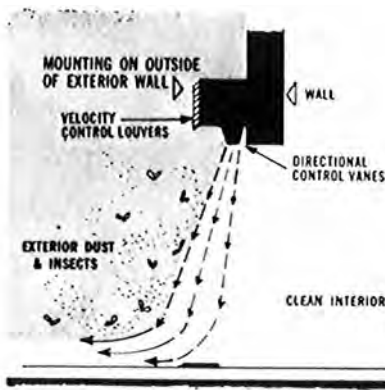
air curtain or air door
