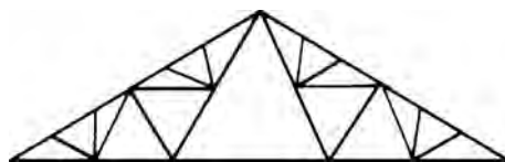
fan Fink truss
