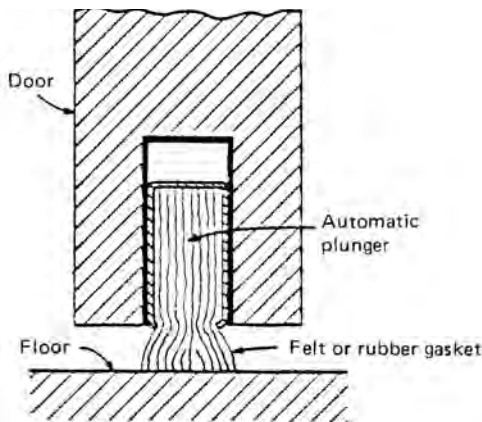
automatic door bottom
