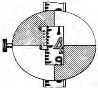
rod target
