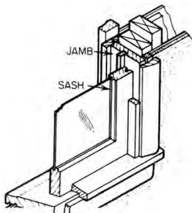
window jamb
