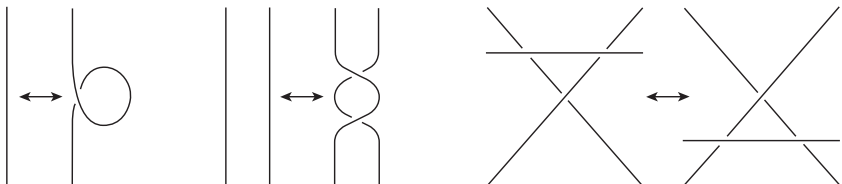
Fig 28 Reidemeister moves.
