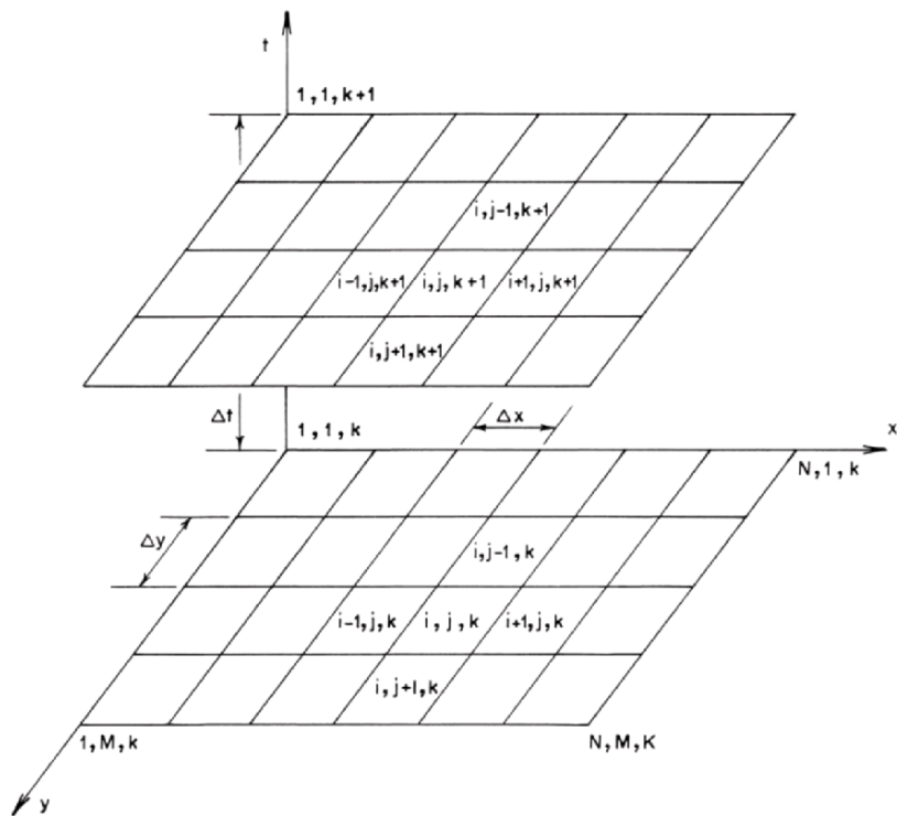
Fig. 15-2. Finite-difference grid
