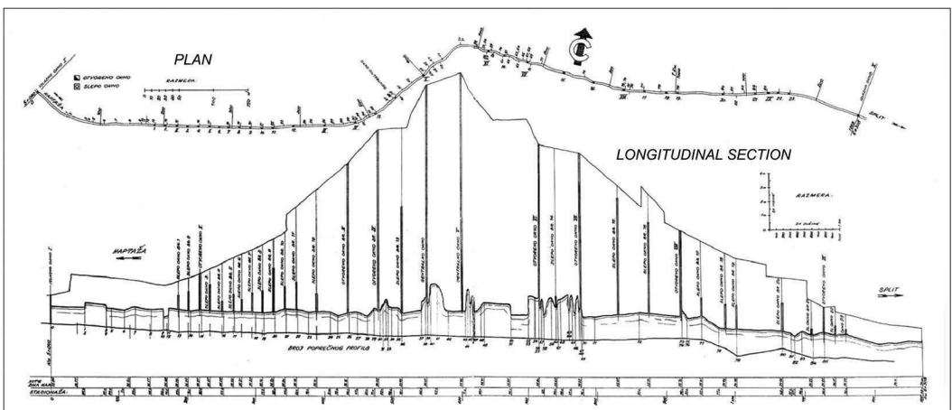
FIGURE 2.9 Plan and longitudinal section of the “Ravne njive” tunnel. (From Katanić, N. and Gojković, M., Građa za proučavanje starih kamenih mostova i akvedukata u Hrvatskoj , JZZSK/RZZZSK SR Hrvatske, Beograd/Zagreb, 1972. With Permission.)
