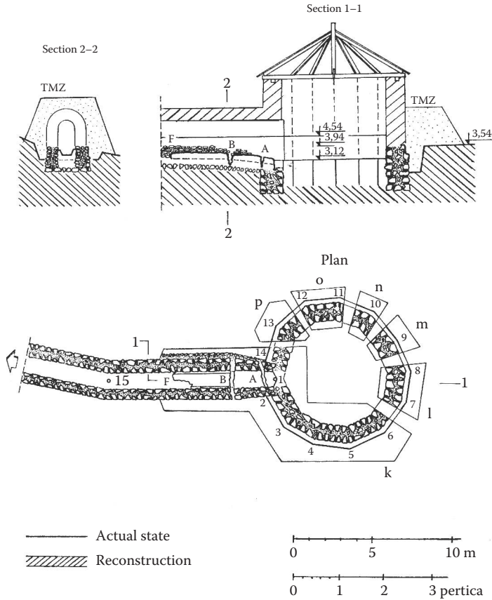
FIGURE 2.4 Polygonal water intake of Aenona aqueduct. (From Ilakovac, B. Rimski akvedukti na području sjeverne Dalmacije, Liber, Zagreb/Arheološki muzej , 1982. With Permission.)
