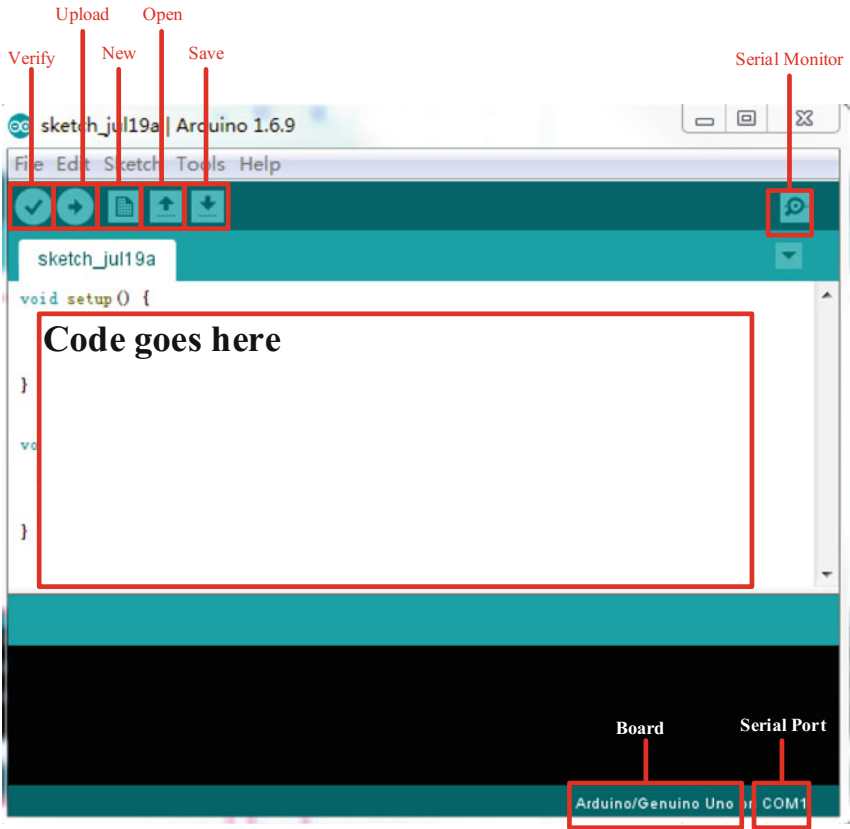
Fig. 1.8 Arduino IDE
