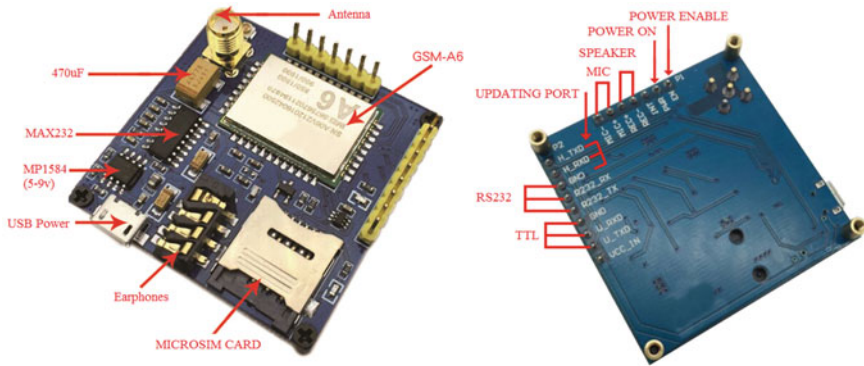
Fig. 5.18 A6 GSM/GPRS module
