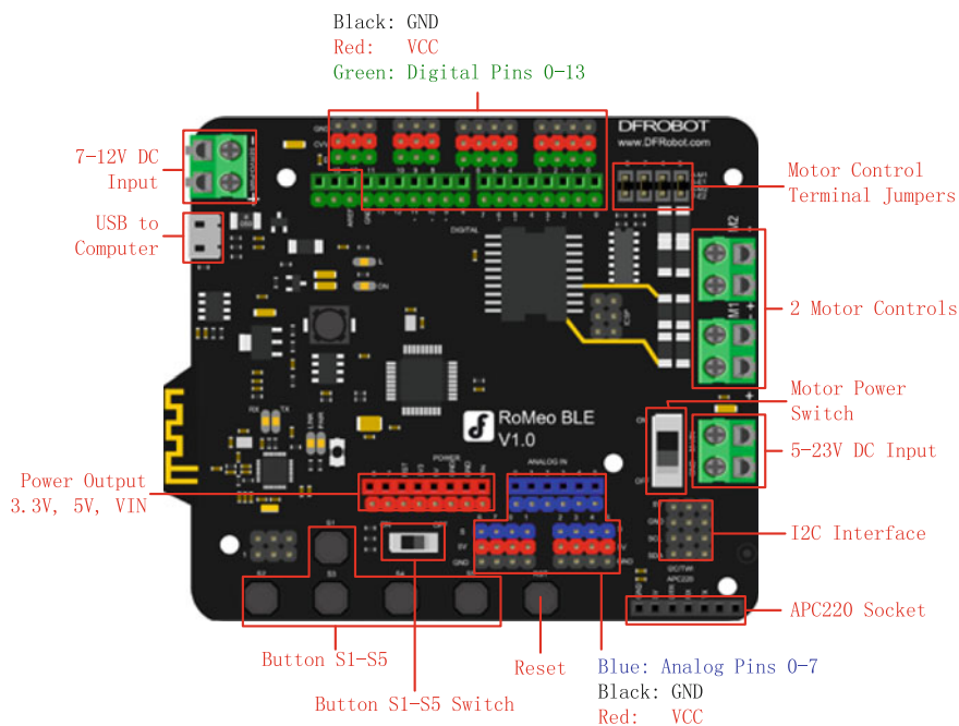
Fig. 1.3 Romeo BLE interface board
