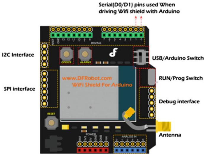
Fig. 5.21 Wi-Fi module
