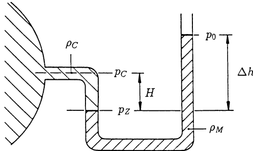
Fig. 5.3. U-tube manometer
