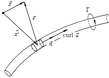
Fig. 4.15. Vortex filament
