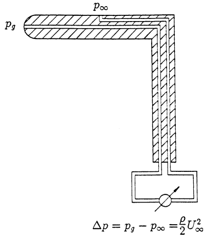
Fig. 10.11. Prandtl tube
