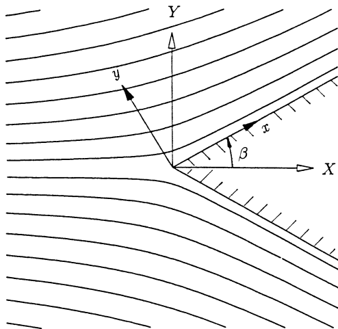
Fig. 12.4. Wedge flow
