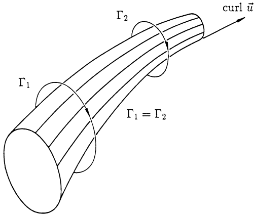
Fig. 4.11. Vortex-tube
