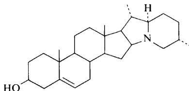
(27)
