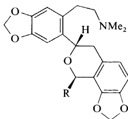
(177)
