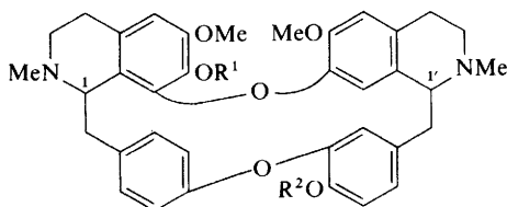
(194)
