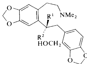
(180)
