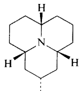
Myrrhine (48)
