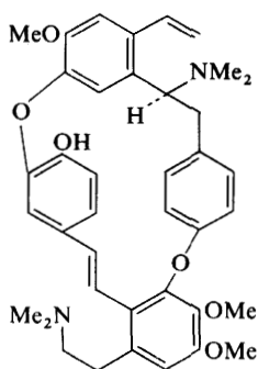
(209)
