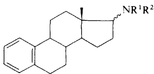
(74)
