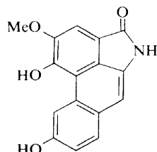
Doryflavine (83) Doryphora sassafras Endlicher 38
