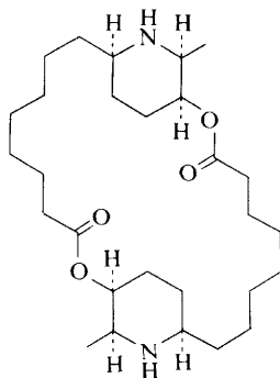
(34)
