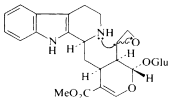
(73)
