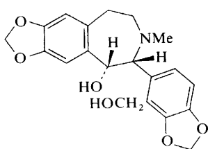
(179)
