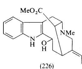
(226)
