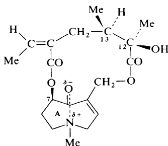
Senkirkinine (24)
