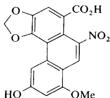
Aristolochic acid-D (71) (aristolochic acid-IVa) Aristolochia indica L. 84 A. clematitis L. 88
