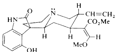
Isotrotundifoleine (85)
