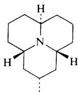
Precoccinelline (46)
