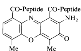
(181)
