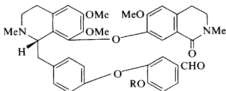
(195)
