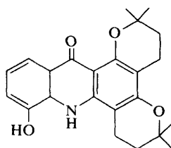
(27)
