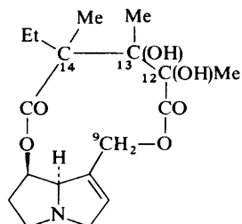
Crotalarine (17)
