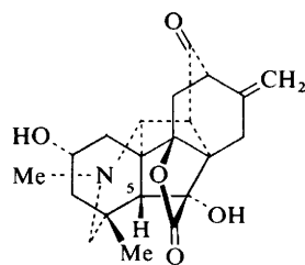
Miyaconine (44)
