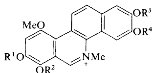
(146)
