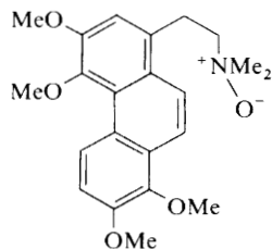
(93)
