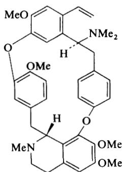
(208)
