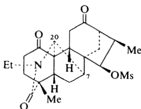
(59)
