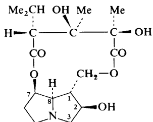
Croalbidine (1)
