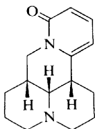
Sophoramine (1)
