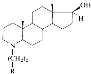
(75) R = NH 2 (76) R = NHC(NH 2 )=NH
