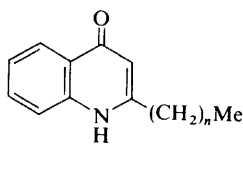
(5)
