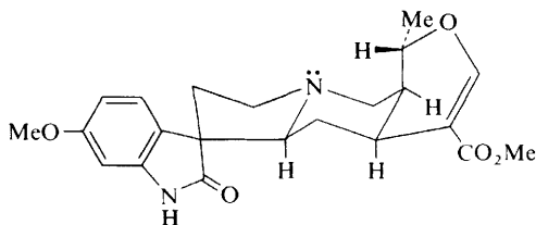
Caboxine A (79)
