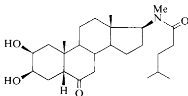
(80)
