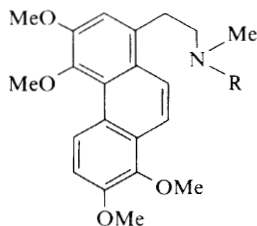
(91) R = Me (92) R = H
