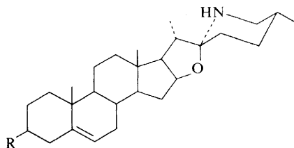
(1) R = OH
