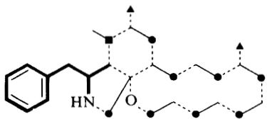
(188)
