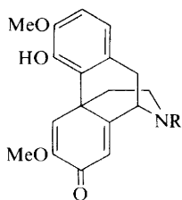
(85)
