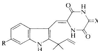
Neoechinulin B (20) R = H, X = CH 2 Neoechinulin C (21) R = CH 2 CH=CMe 2 , X = CH 2 Neoechinulin (22) R = CH 2 CH=CMe 2 , X = O
