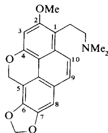
(97)
