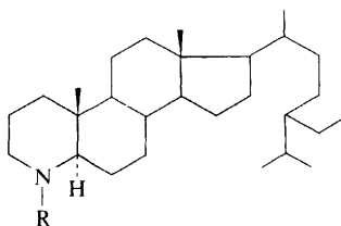
(77) a; R = H b; R = Me
