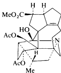
Yuzurimine (3)
