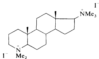
(79)
