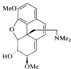
(80)
