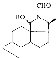
(51)
