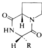
(136) R = Bu i (137) R = CH 2 Ph
