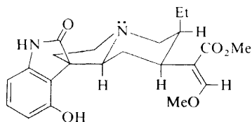
Isomitrafoline (81)
