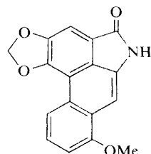
Aristolactam (74) Aristolochia debilis Sieb. et Zucc. 86,87 Aristolochia indica L. 84
