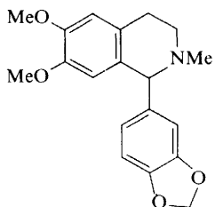
(105)
