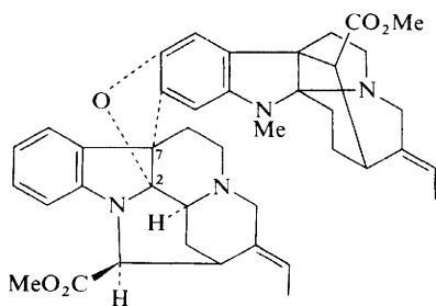
Pleiocorine (228)
