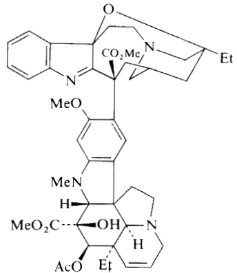
(234)
