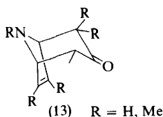
(13) R = H, Me
