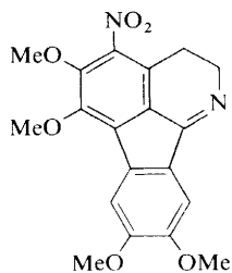
(106)
