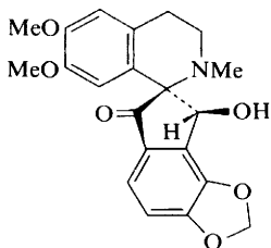
(181)
