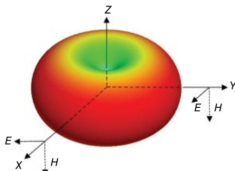
Slot antenna
