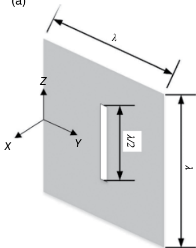
Slot antenna
