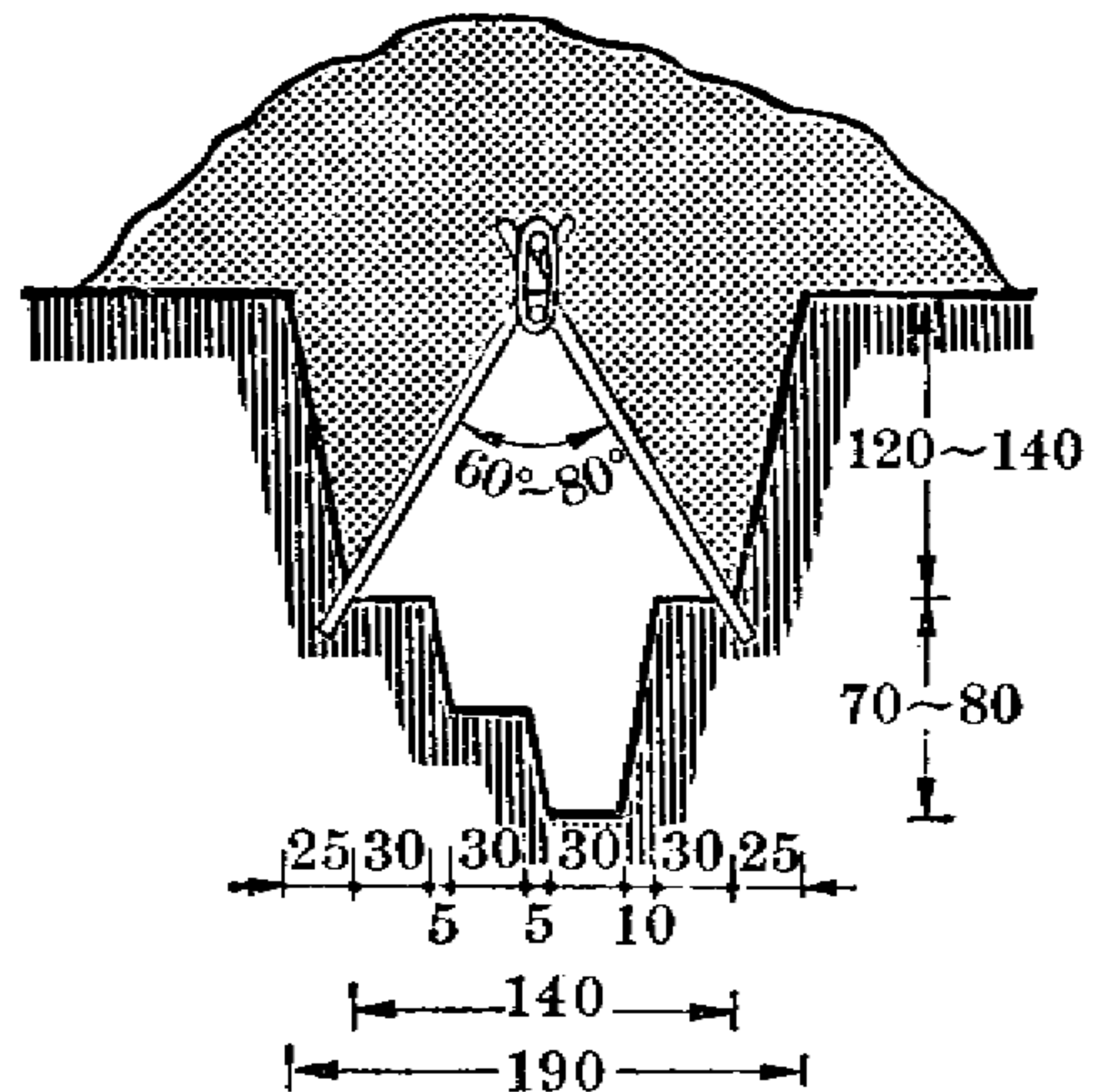
图 3-107 人字形骨架避弹所
