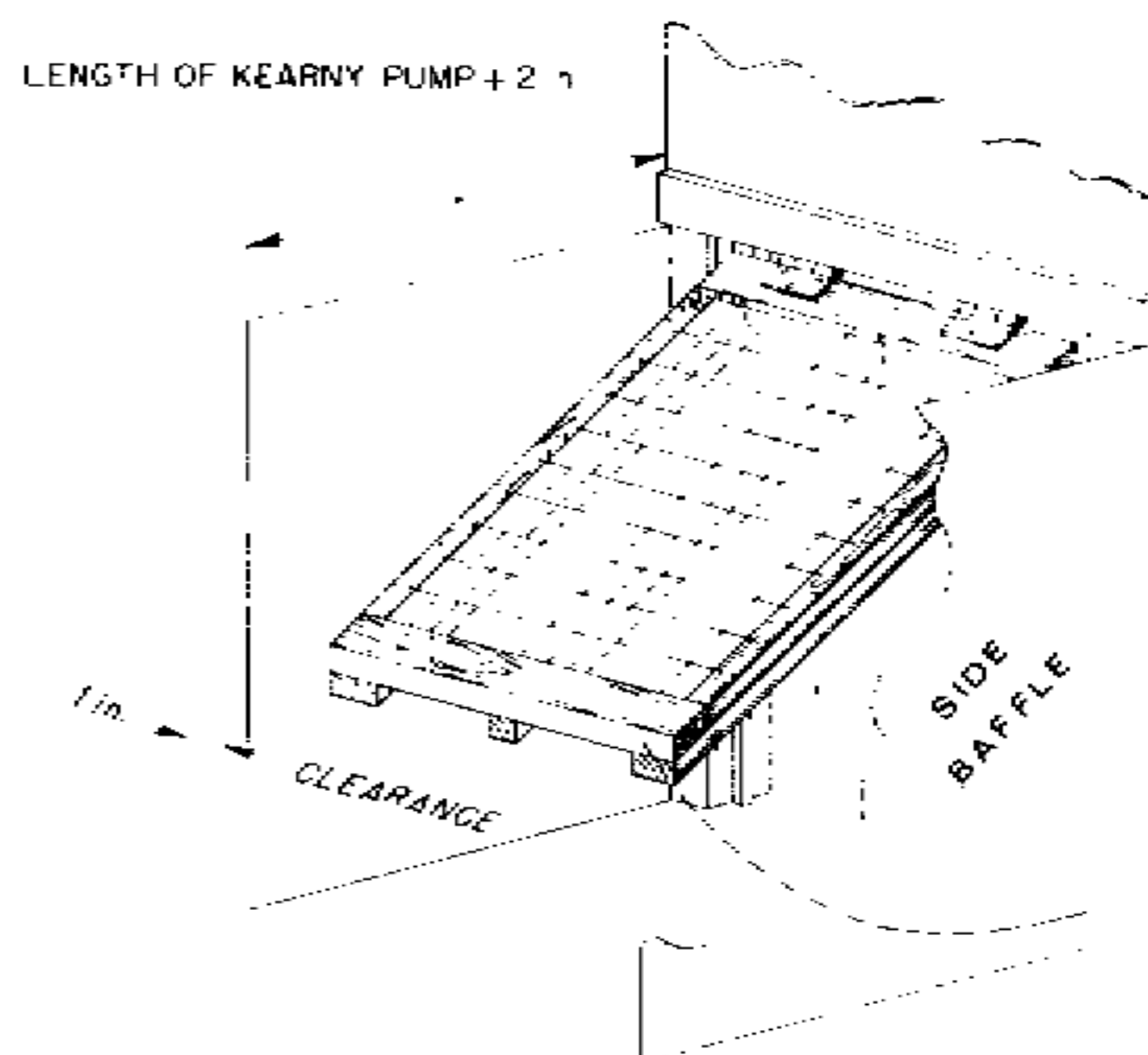
Fig. 25. Side baffles.
