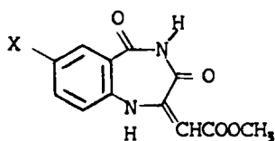
X=Halogen, CH 3 , C 6 H 5 , O
